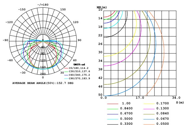
C0等高线平面图 (单位: lx)
