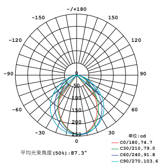
发光强度分布图
