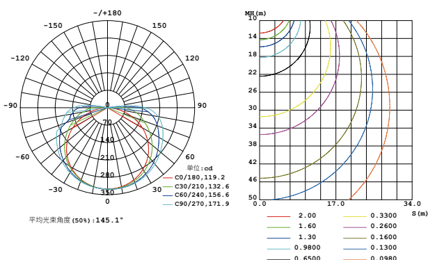
发光强度分布图
