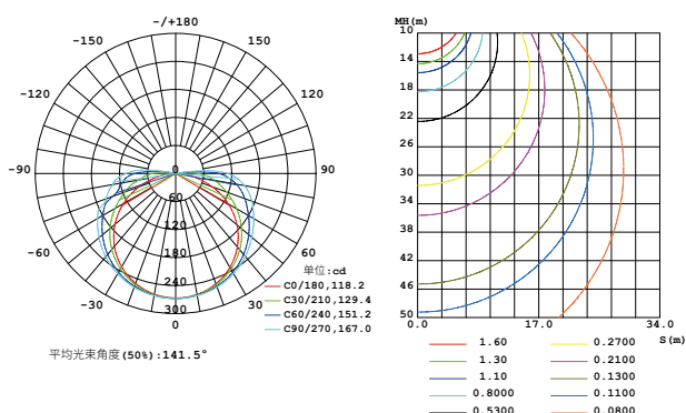
发光强度分布图
