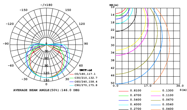
发光强度分布图
