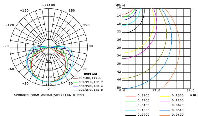
C0等高线平面图 (单位: lx)
