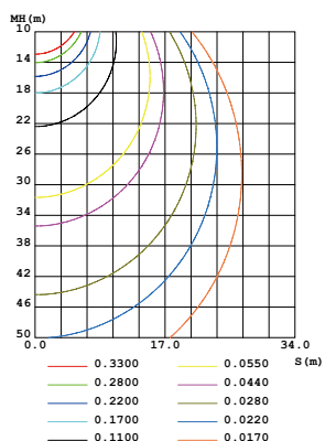
C0等高线平面图 (单位: lx)
