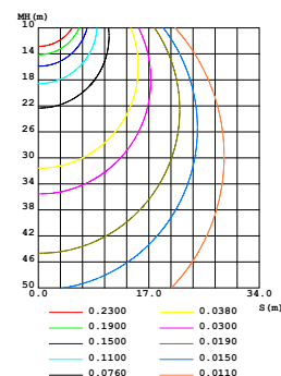
空间等照度曲线(单位:lx)
