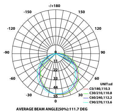
室内灯具配光曲线
