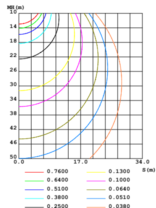
空间等照度曲线(单位:lx)
