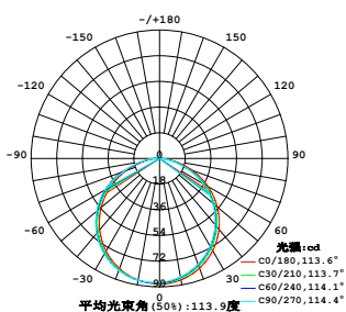
室内灯具配光曲线
