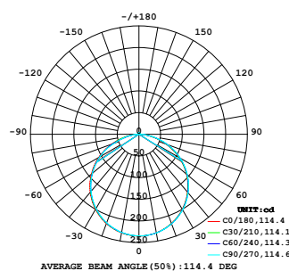
室内灯具配光曲线
