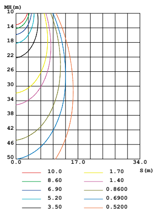
C0等高线平面图 (单位: lx)
