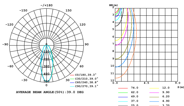
室内灯具配光曲线
