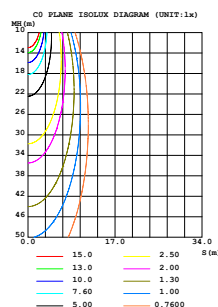
空间等照度曲线(单位:lx)
