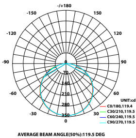
室内灯具配光曲线
