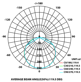
室内灯具配光曲线
