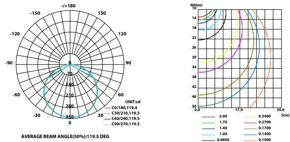
空间等照度曲线(单位:lx)
