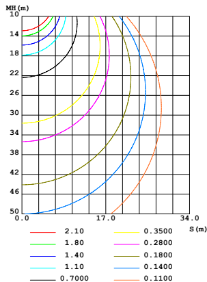
空间等照度曲线(单位:lx)
