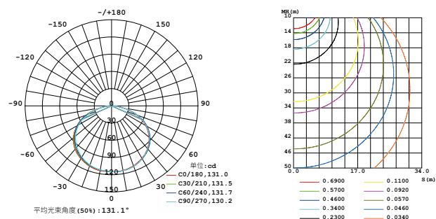
发光强度分布图
