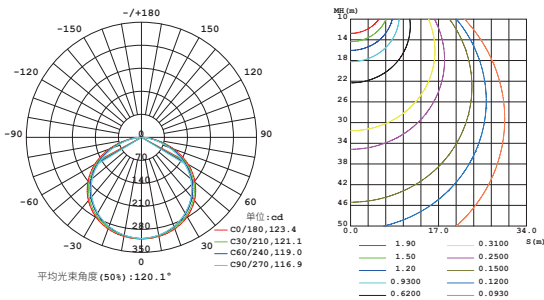
发光强度分布图 C0等高线平面图（单位：lx）
