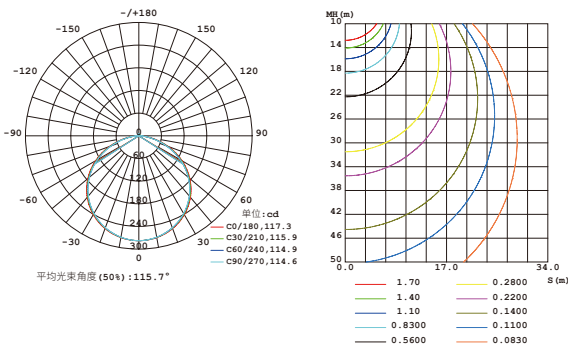
发光强度分布图
