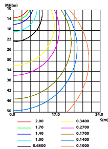
空间等照度曲线(单位:lx)
