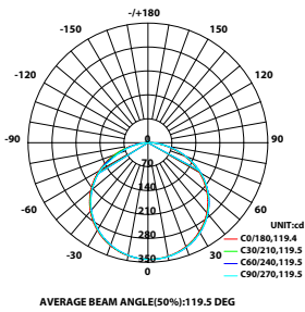
室内灯具配光曲线
